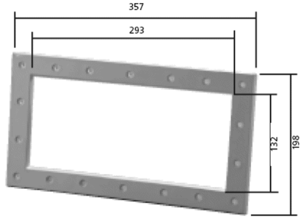
miniskimmer szeroki
